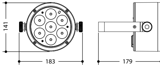
Disegno tecnico
