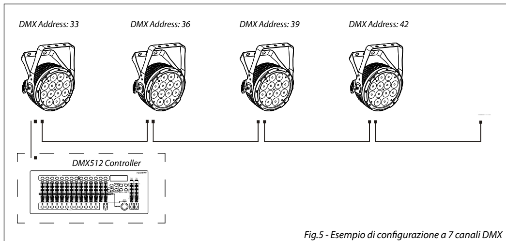
Fig.5 - Esempio di configurazione a 7 canali DMX
