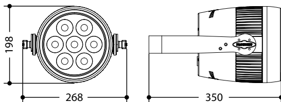
Disegno tecnico
