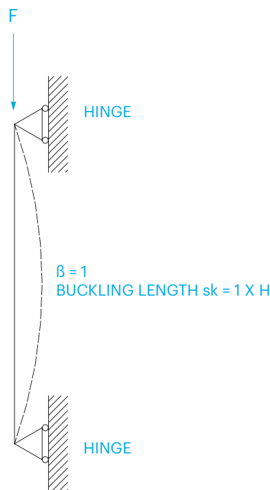
EULER 2E
