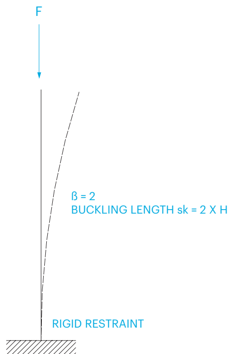
EULER 1E
