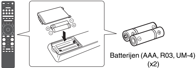
Afstandsbediening
